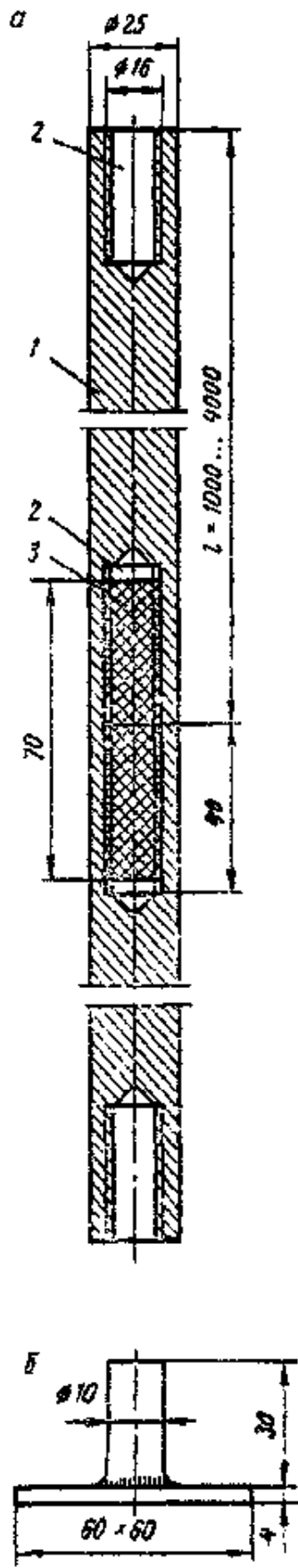
Рис. 40. Соединение домкратных стержней:
