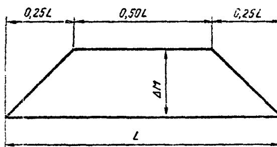
Рис. 1. Эпюра момента \Delta M от волновой нагрузки
