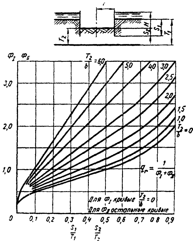
Рис. 2. График для определения q_r = f\left(\frac{S_1}{T_1}; \frac{S_2}{T_2}\right) в случае близкого расположения водоупорного слоя ( \Phi_1 определяется в функции \frac{S_1}{T_1} ; \Phi_2 – в функции \frac{S_2}{T_2} )
