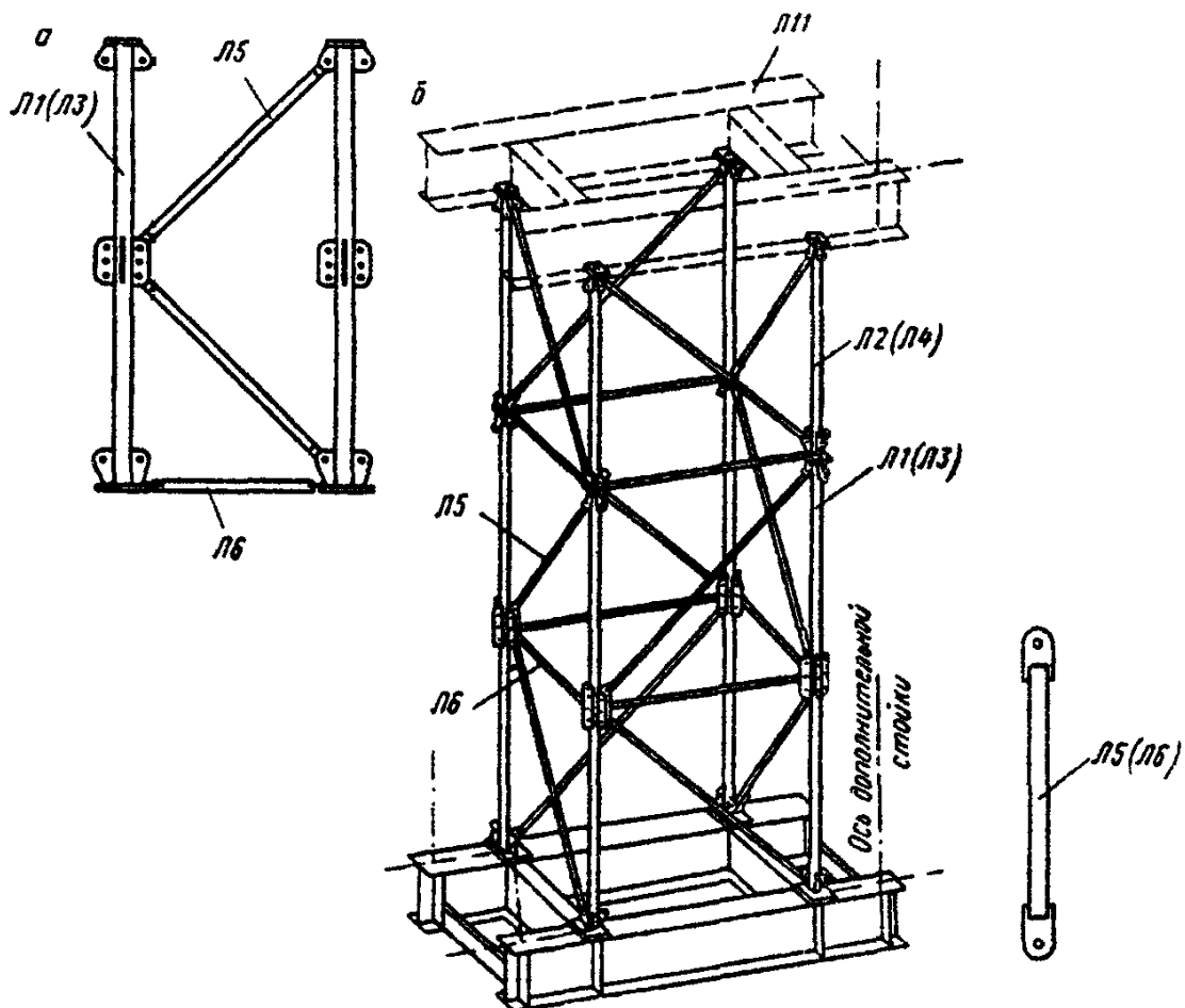
Рис. 1. Схема сборки опоры из элементов МИК-С:
