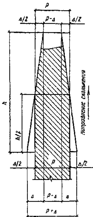
Рис. 39. Схема наклона щитов скользящей опалубки
