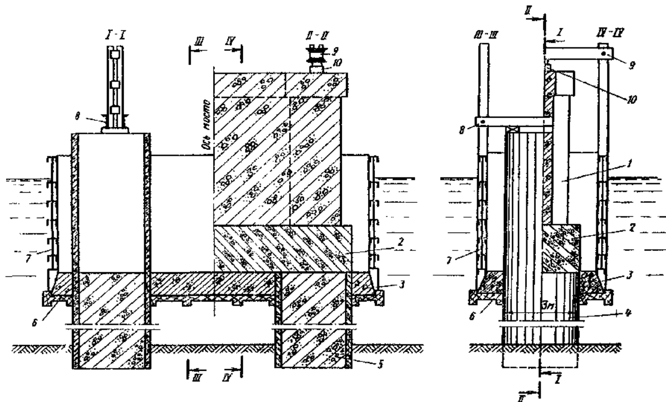
Рис. 13. Металлическое щитовое ограждение ростверка:
