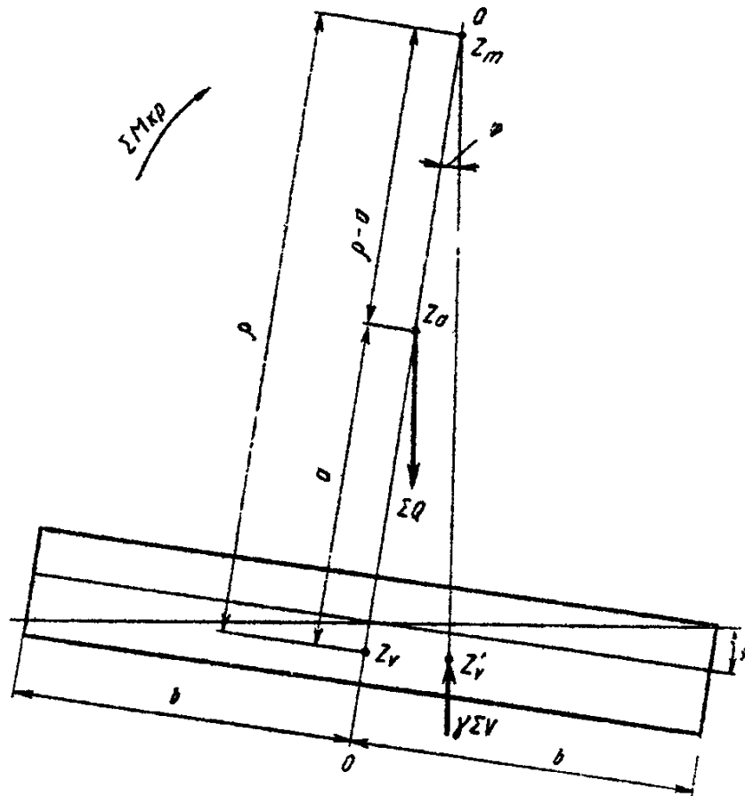
Рис. 56. Схема определения остойчивости плавучей опоры
