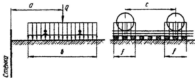
Рис. 4. К определению эквивалентной нагрузки от двухрельсовой тележки на призме обрушения
