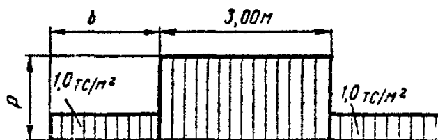
Рис. 1. Вертикальная нагрузка на призме обрушения от автотранспорта
