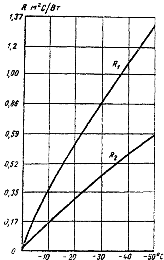
Рис. 37. Кривые зависимости оптимального термического сопротивления боковых поверхностей опоры R_1 (в \text{м}^2\text{С}/\text{Вт} ) от расчетной температуры наружного воздуха, ^{\circ}\text{С} ( R_1 - для торцовых поверхностей и боковых частей поверхности, прилегающих на 2 м к углам опоры; R_2 - для остальных частей боковых поверхностей)
