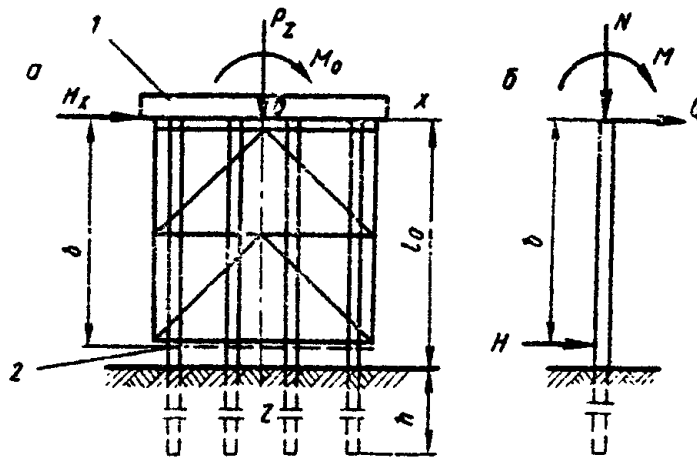
Рис. 2. К расчету свайных фундаментов, усиленных каркасом:
