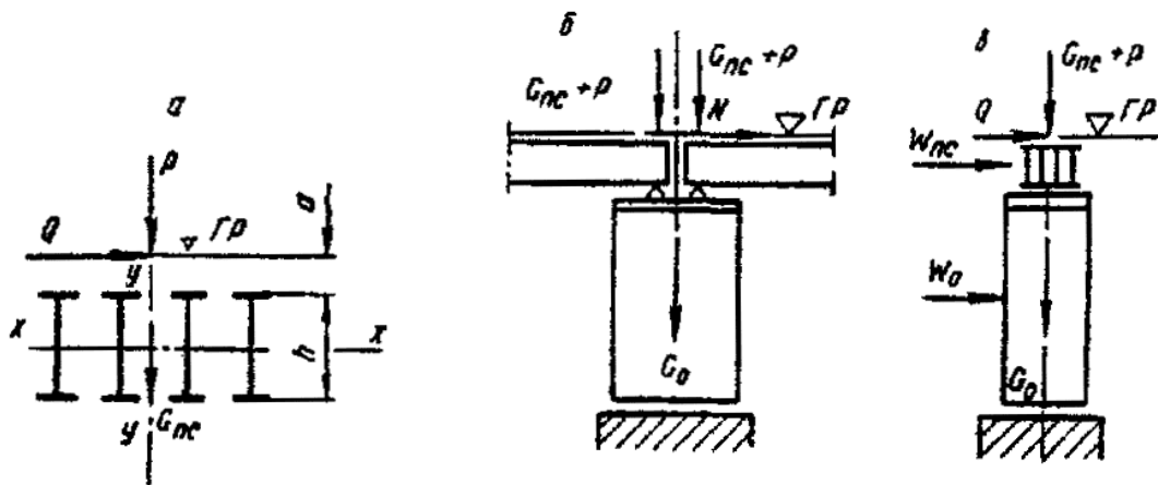
Рис. 1. Схемы приложения нагрузок в подкрановых эстакадах:
