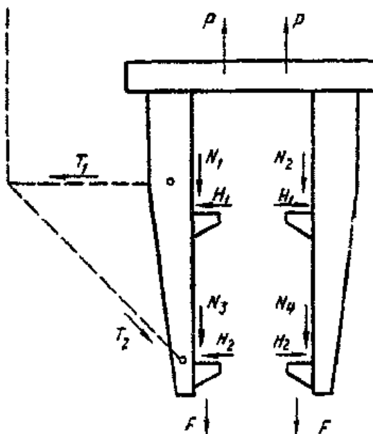
Рис. 41. Нагрузки, действующие на скользящую опалубку:
