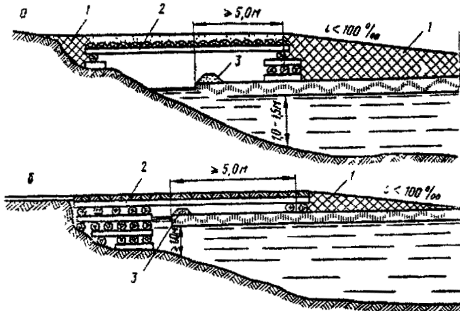
Рис. 4. Сопряжение ледовой дороги с берегом:
