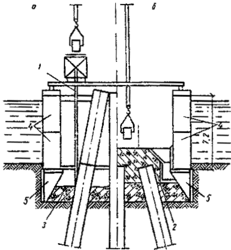
Рис. 12. Бездонный ящик из понтонов КС:
