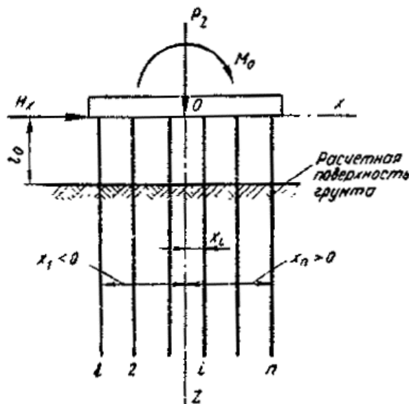
Рис. 61. Расчетная схема фундамента из вертикальных свай
