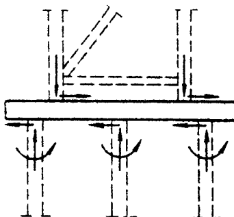
Рис. 63 Схема для расчета конструкции, объединяющей головы свай
