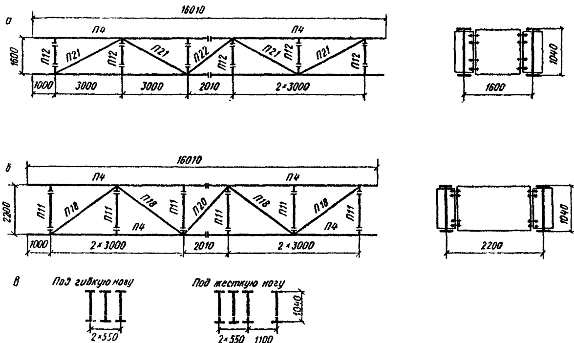
Рис. 1. Примерные монтажные схемы пакетных пролетных строений:
