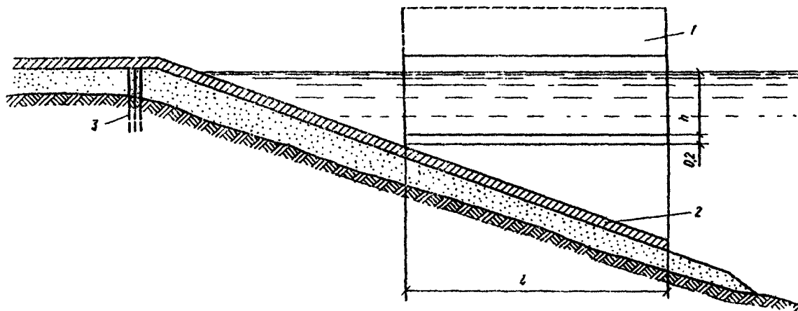
Рис. 3. Схема для расчета длины наклонной части стапеля:
