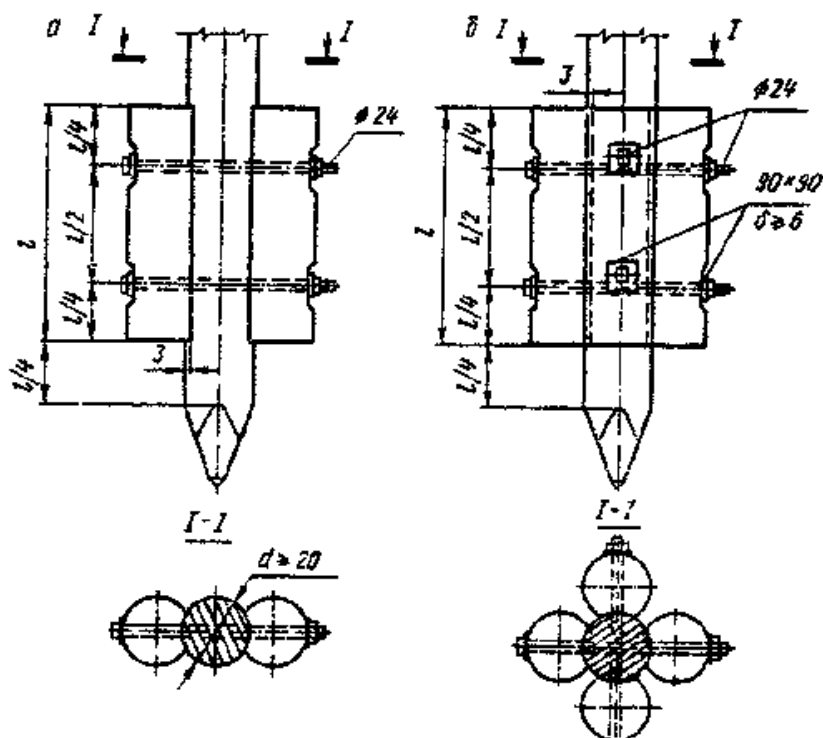
Рис. 60. Забивные деревянные сваи с уширенной пятой:
