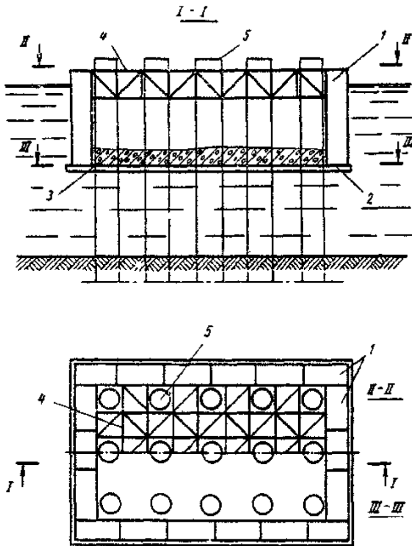
Рис. 14. Перегородка из понтонов КС:
