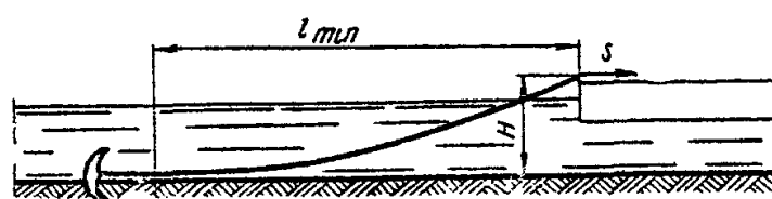
Рис. 57. Схема определения длины якорного каната
