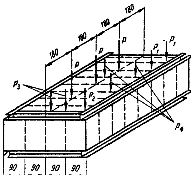
Рис. 1. Схема универсального понтона КС
