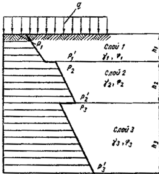
Рис. 8. К определению активного давления грунта из нескольких слоев песка или супеси на стенку ограждения
