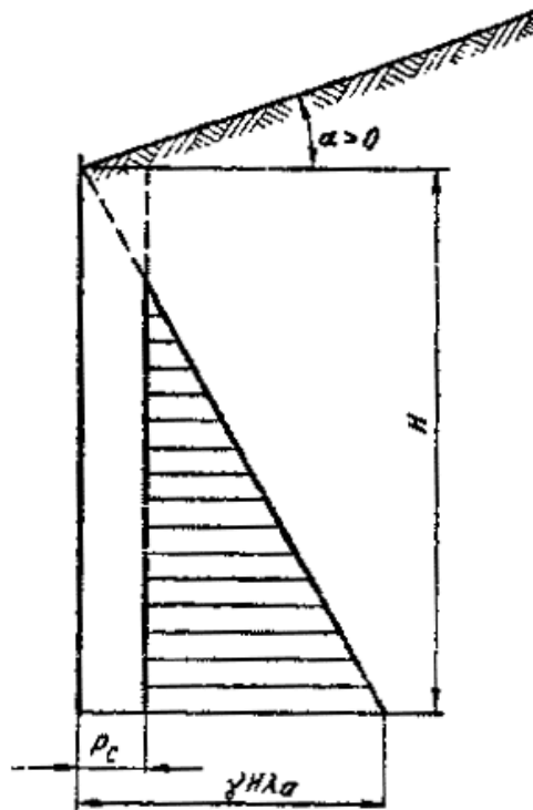
Рис. 9. К определению активного давления суглинка или глины
