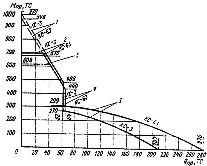
Рис. 3. График предельных усилий на понтон при изгибе в плоскости палубы:
