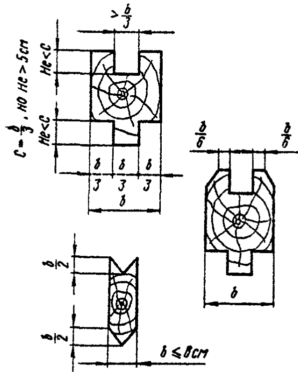
Рис. 24. Поперечное сечение деревянного шпунта
