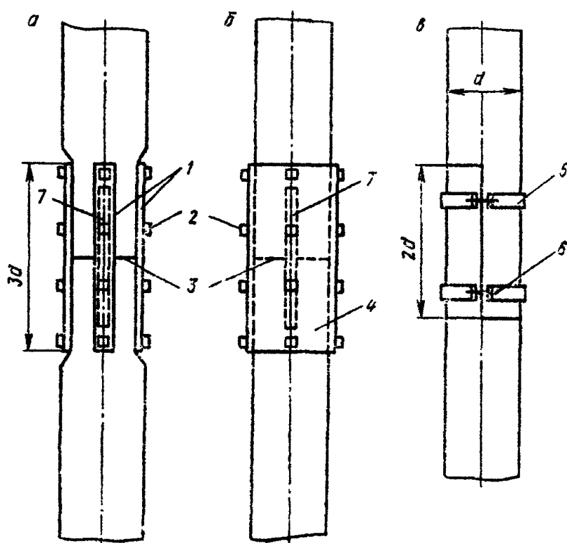
Рис. 59. Стык деревянных свай:
