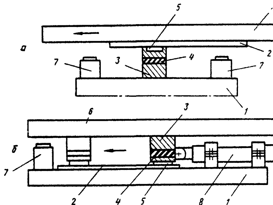
Рис. 50. Устройства скольжения циклического действия:
