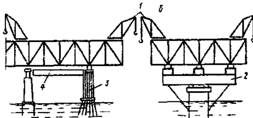
Рис. 42. Опорные устройства для уравновешенной сборки:
