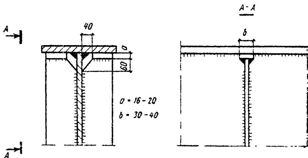
Рис. 64. Примыкание ребер жесткости к поясам балок
