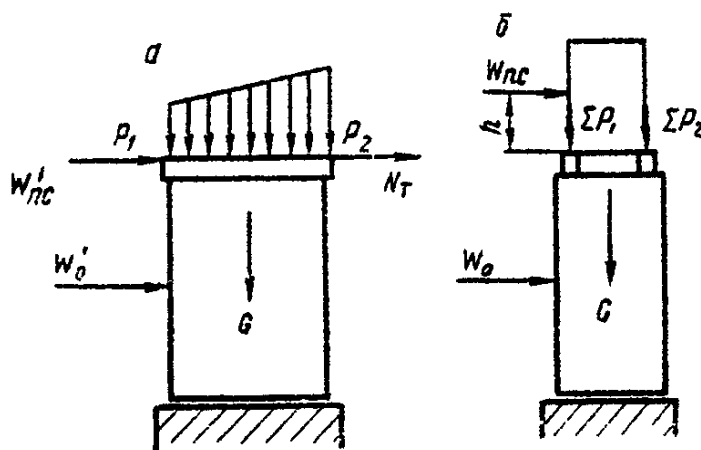
Рис. 45. Схема приложения нагрузок к перекаточной опоре:
