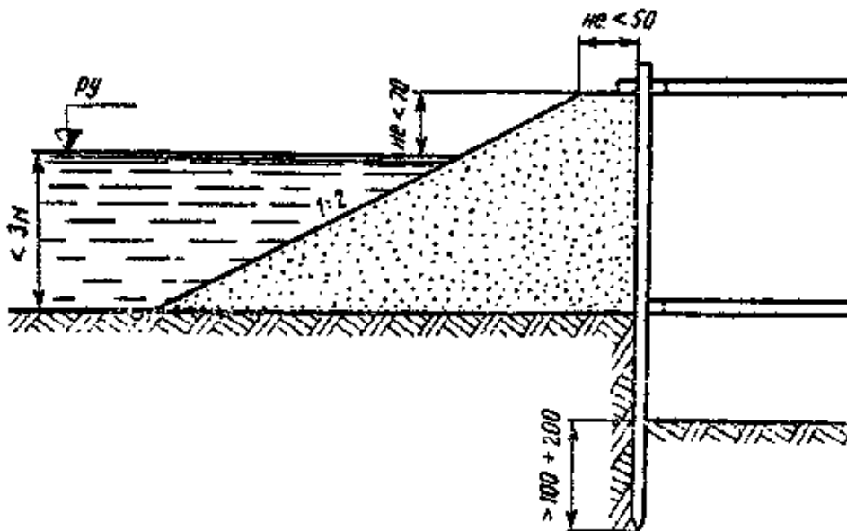
Рис. 10. Шпунтовая однорядная перемишка с односторонней отсыпкой грунта
