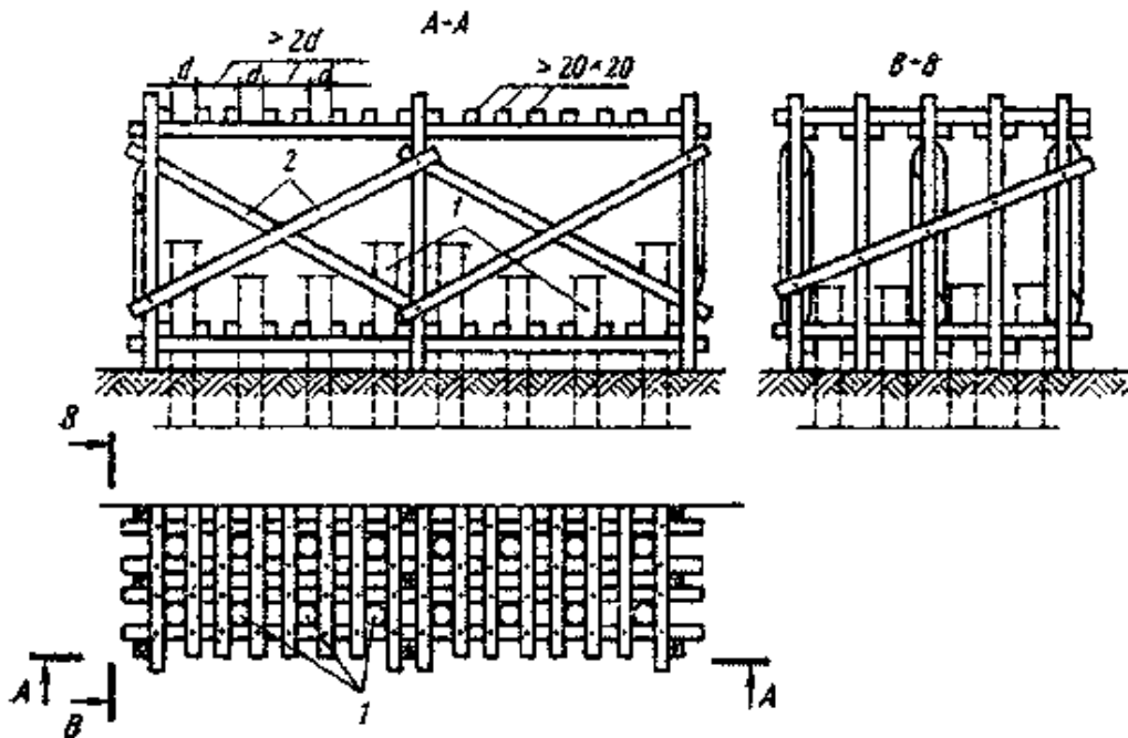
Рис. 28. Направляющий каркас из деревянных элементов:
