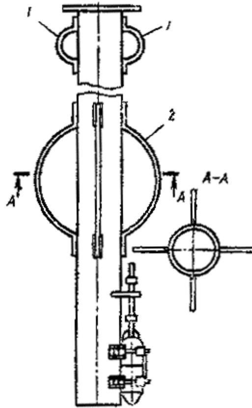
Рис. 31. Фиксирующие и направляющие устройства на бетонолитной трубе:
