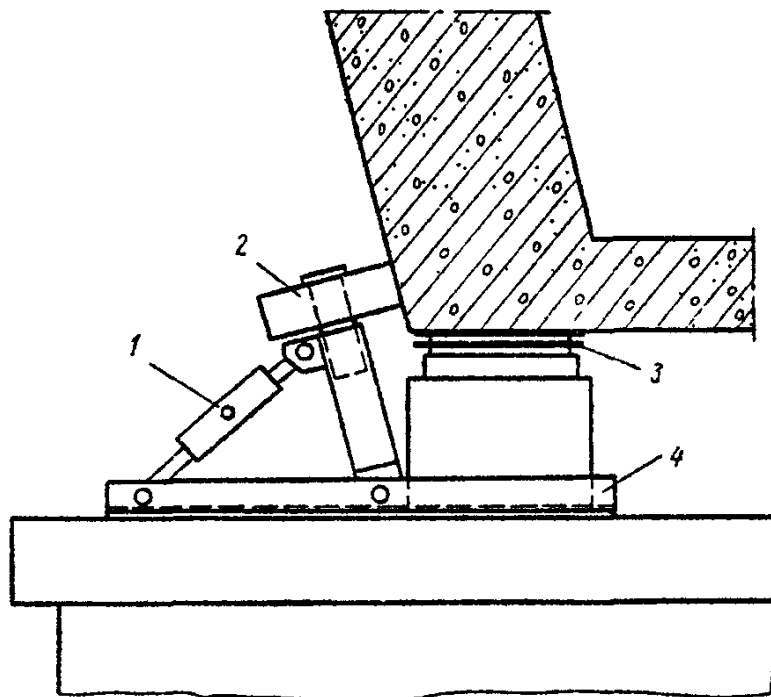
Рис. 53. Направляющее устройство:
