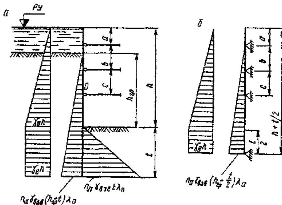
Рис. 22. Схемы расчета шпунтовых ограждений с двумя и более ярусами креплений:
