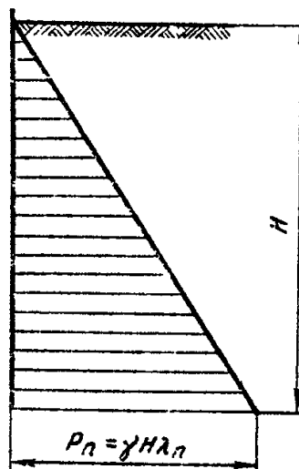
Рис. 10. Эпюра пассивного давления песка или супеси на стенку ограждения
