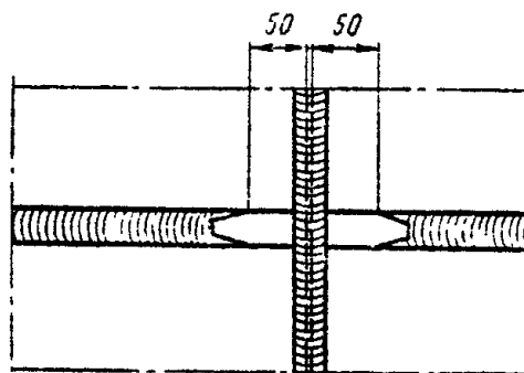
Рис. 66. Пересечение стыковых швов
