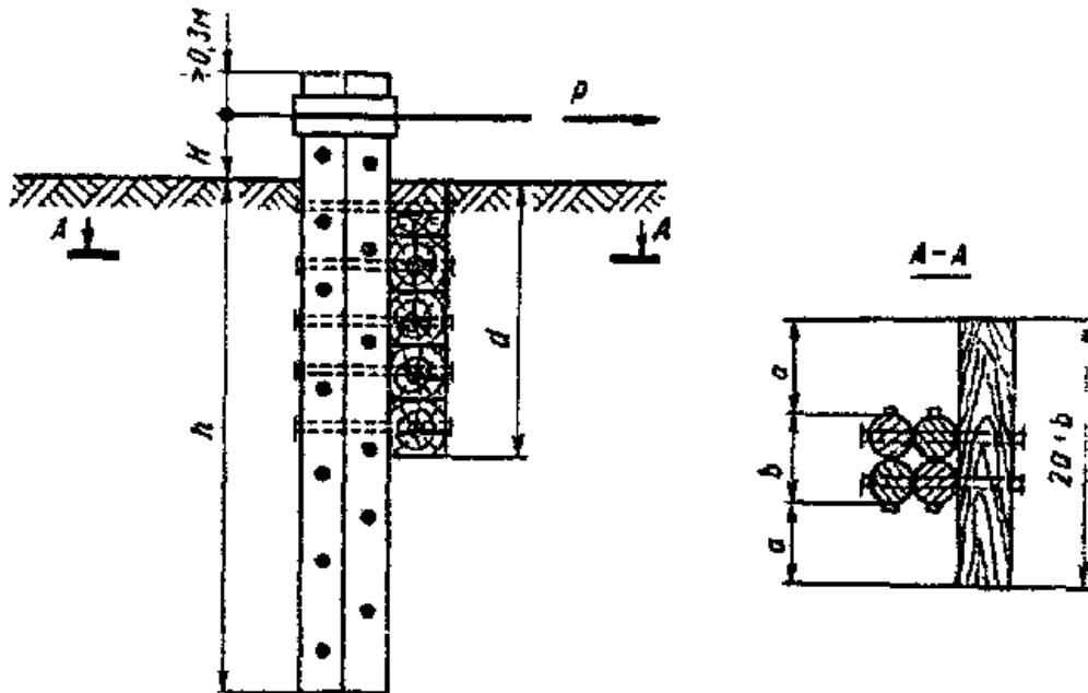
Рис. 8. Свайный якорь
