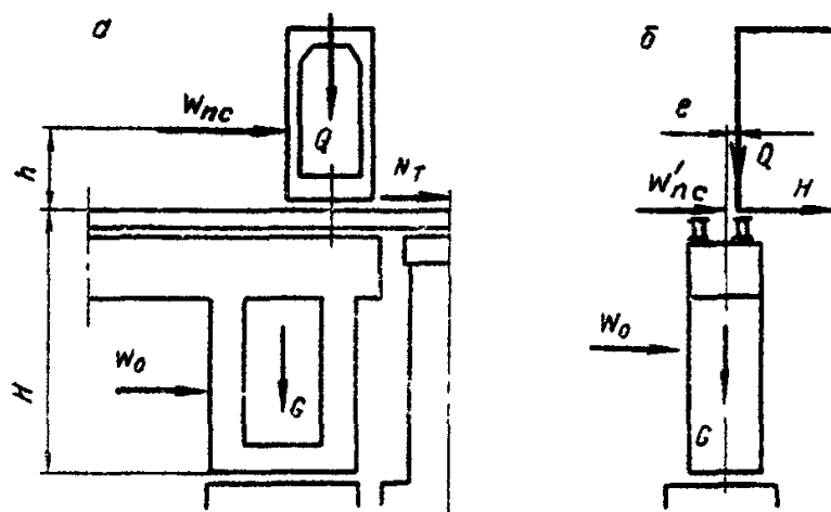
Рис. 47. Схемы приложения нагрузок к пирсам:
