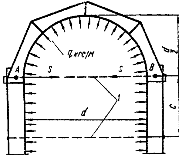
Рис. 35. Расчетная схема кружальных ребер опалубки опор:
