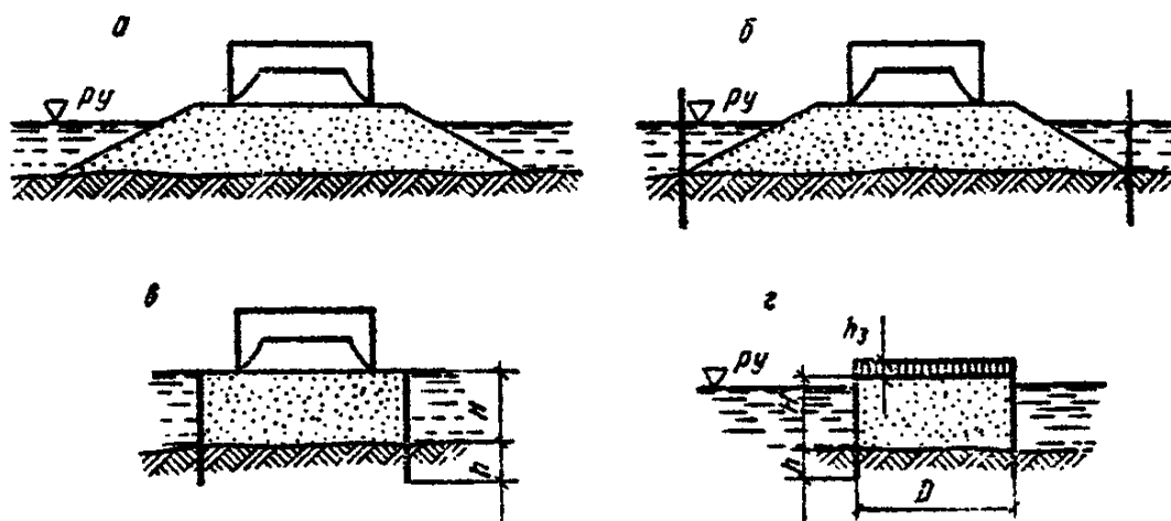
Рис. 26. Схемы искусственных островков:
