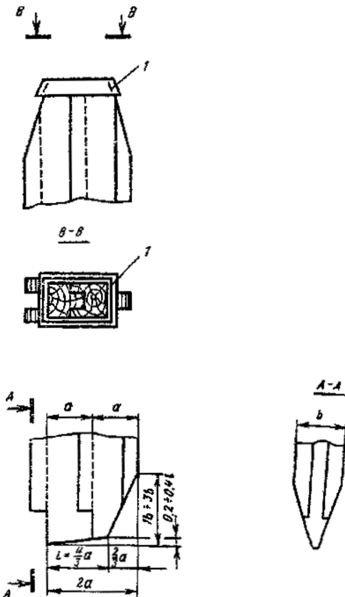
Рис. 25. Конструкция деревянных шпунтовых свай:
