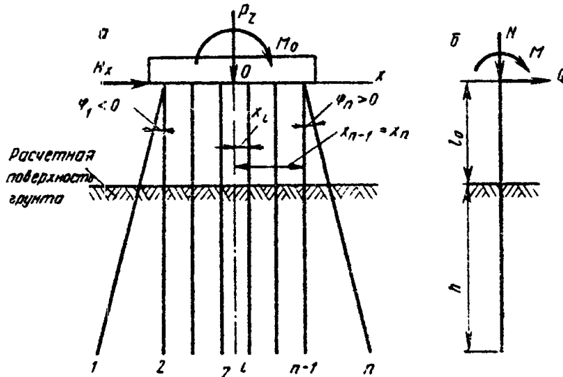
Рис. 1. К расчету свайных фундаментов, не усиленных каркасом:
