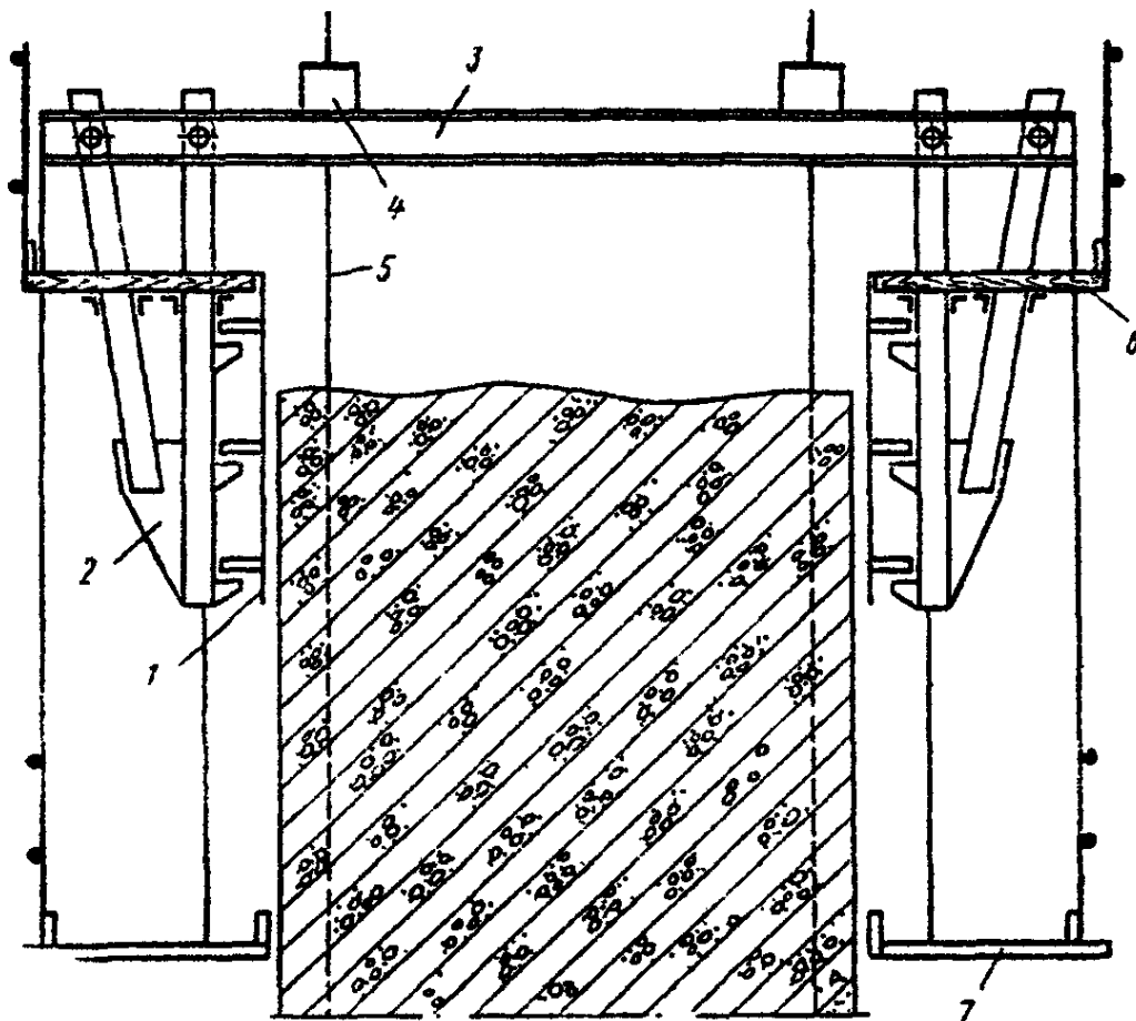
Рис. 38. Стержневая скользящая опалубка
