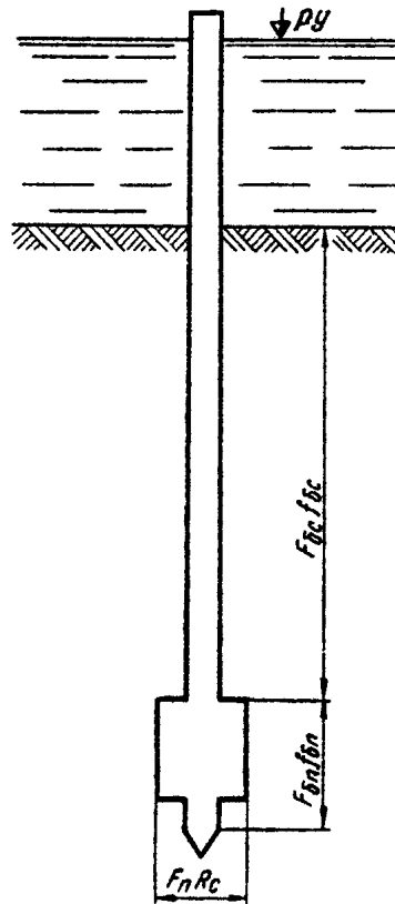
Рис. 58. Расчетная схема определения несущей способности забивкой сваи с уширенной пятой
