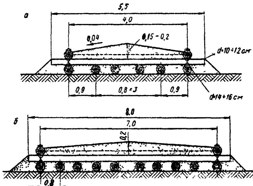
Рис. 7. Типы лежнево-сланевой дороги:
