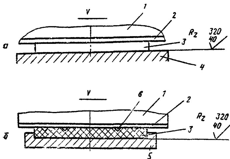
Рис. 51. Расположение в устройствах скольжения антифрикционных прокладок:
