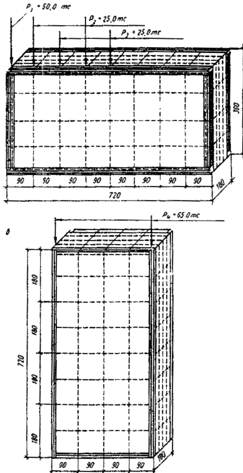
Рис. 4. Схема предельных нагрузок на понтон при использовании его в конструкциях подмостей: a - на узлы борта; б - на узлы торца P_1=50 тс при условии постановки металлических вкладышей в горизонтальные коробки в месте опирания
