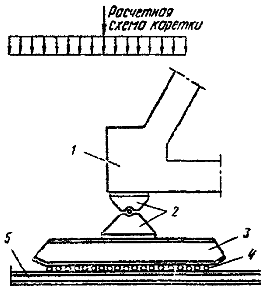
Рис. 54. Опирание узла пролетного строения на накаточные пути при продольной подвижке на плаву:
