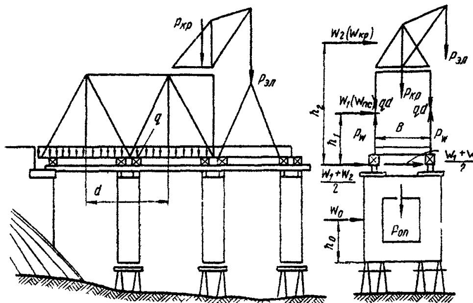
Рис. 44. Расчетная схема сборочных подмостей
