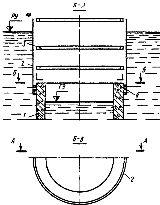
Рис. 15. Стальное ограждение верхней части круглого колодца:
