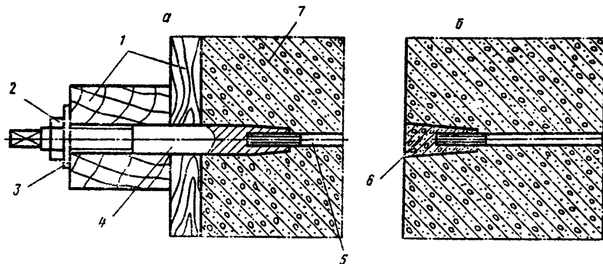
Рис. 34. Тяжи со съемными наконечниками:
