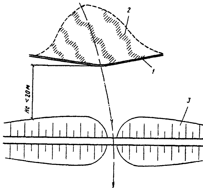
Рис. 6. Противоналедные устройства из заборов или переносных щитов:
