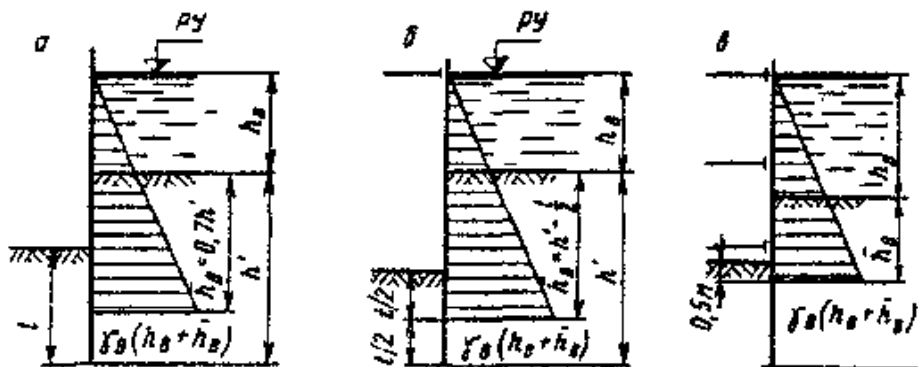
Рис. 16. Схемы для определения глубины проникания воды между шпунтовой стенкой и водонепроницаемым грунтом:
