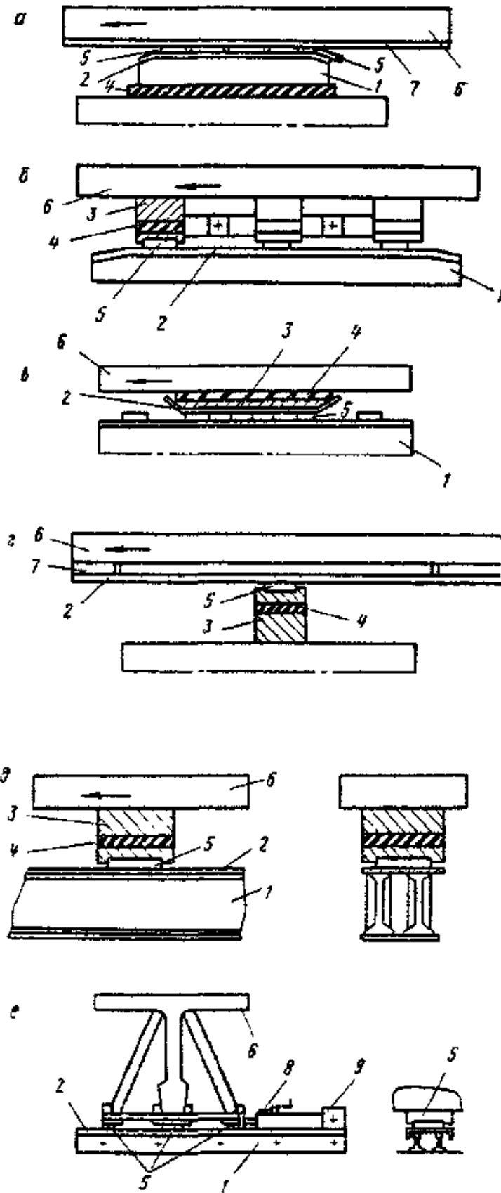
Рис. 49. Устройства скольжения непрерывного действия:
