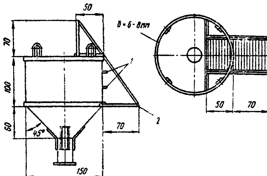
Рис. 30. Конструкция приемной воронки объемом 2 м 3 с площадками:
